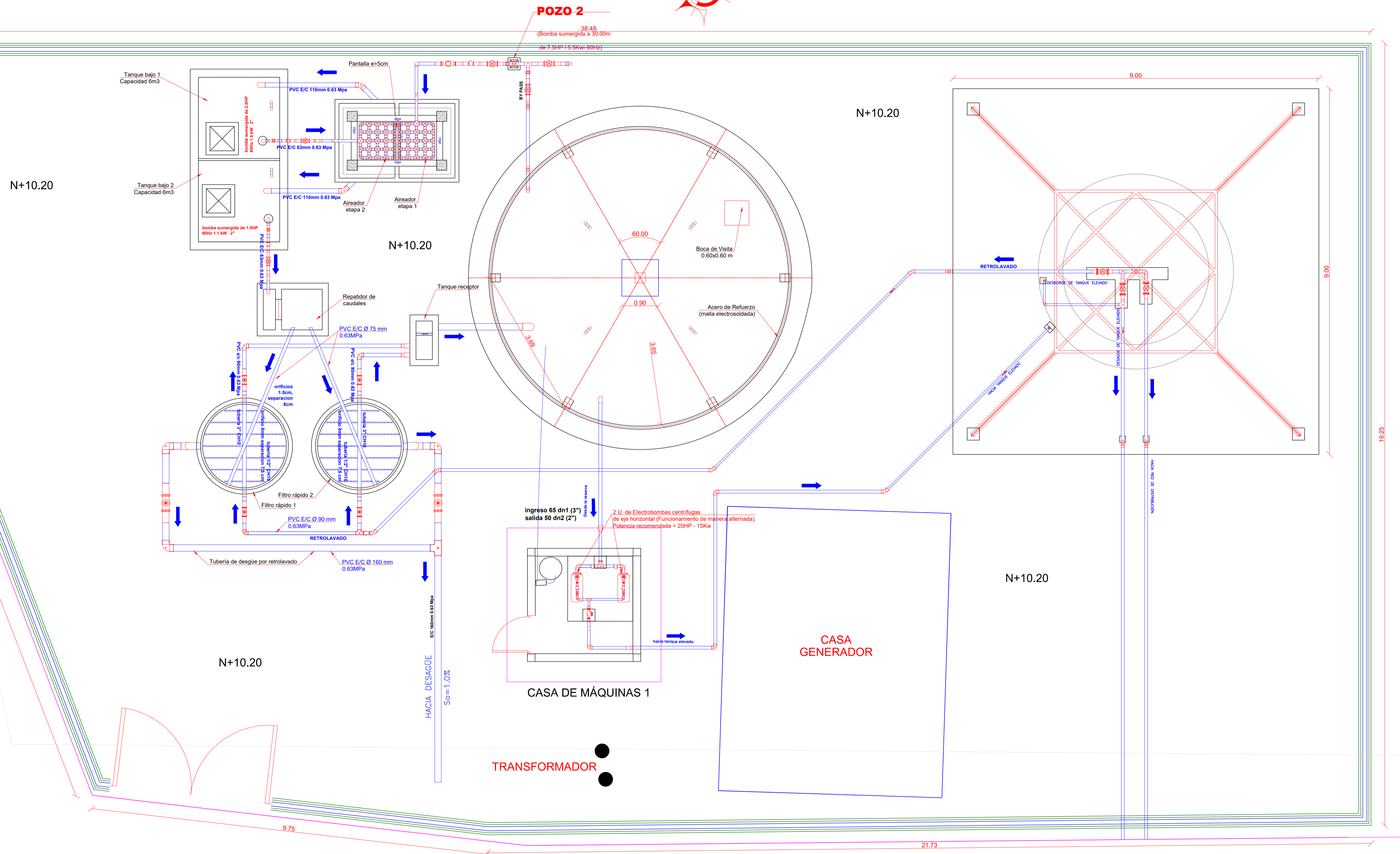
IMPLANTACIÓN PLANTA DE POTABILIZACIÓN DE AGUA Escala: 1:50
